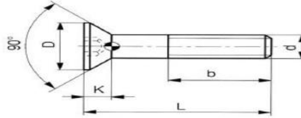
HAVŞA BAŞLI İMBUS CİVATA ÖLÇÜLERİ
